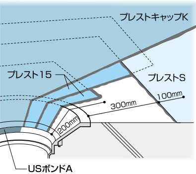
露出工法
