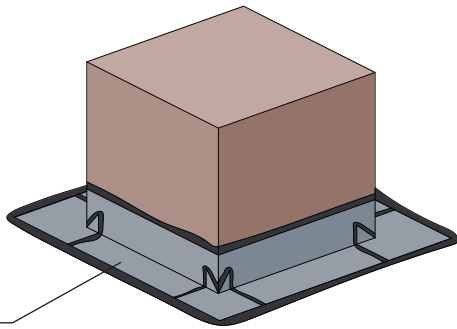
増張りアスリードルーフ W=300
