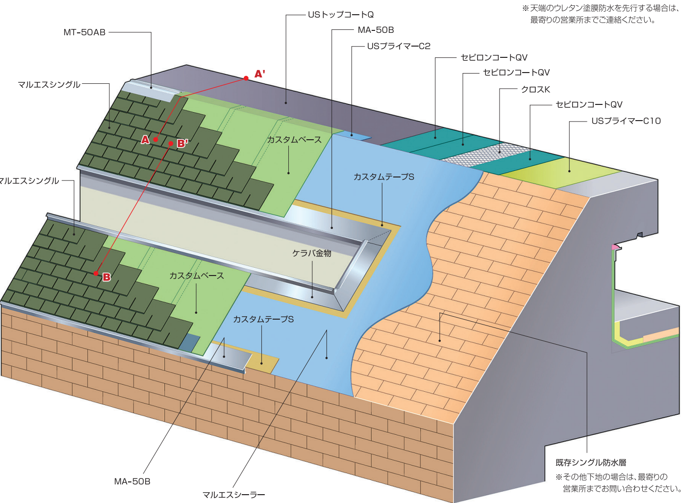
斜壁 納まり図
