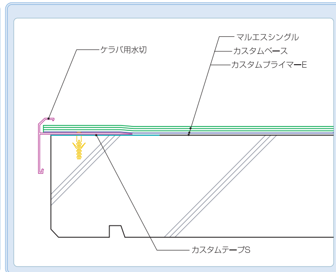
ケラバ部（非断熱）
