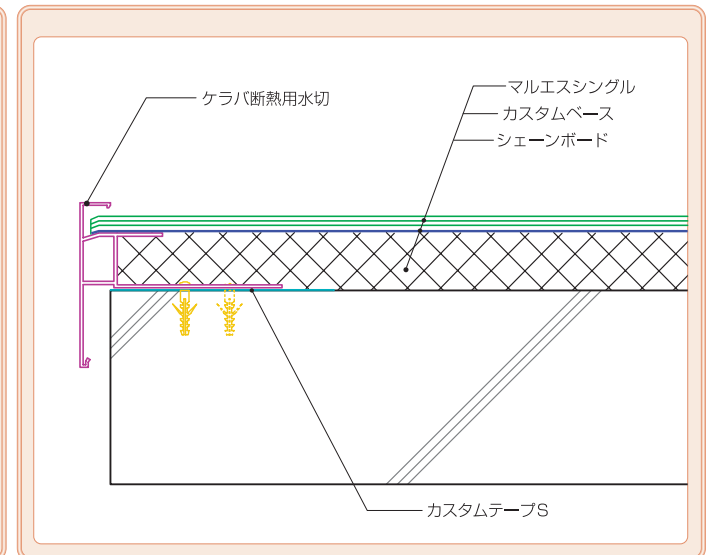
ケラバ部（断熱）
