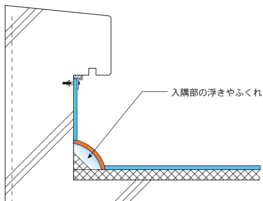
入隅部分に浮きや膨れがある場合
