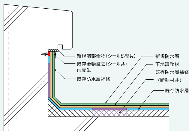
■ 劣化ランクA～B 改修後
