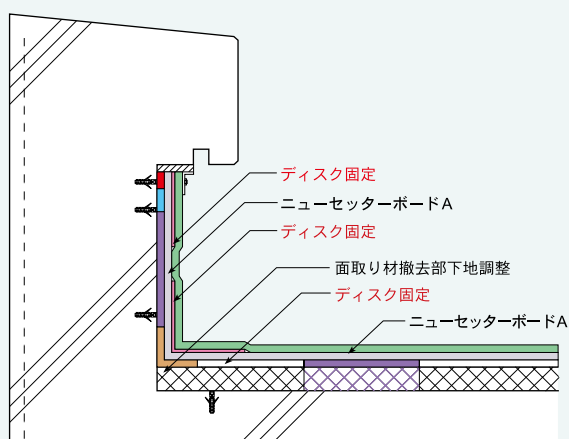
■ 劣化ランクC ニューセッターボードAを用いて下地調整した場合の改修後
