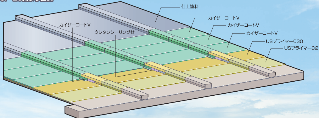
KMCF-20納まり図例
