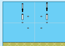
④スペーサーを差し込み、エポキシ樹脂を注入してプラグを差し込む
