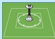
⑧押えキャップ・ナット・天板を取り付ける
