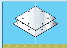
③テンプレート6で穴をあける
