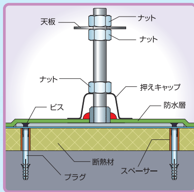
①断熱材の施工
