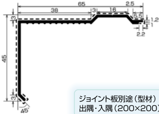
MT-42BU
