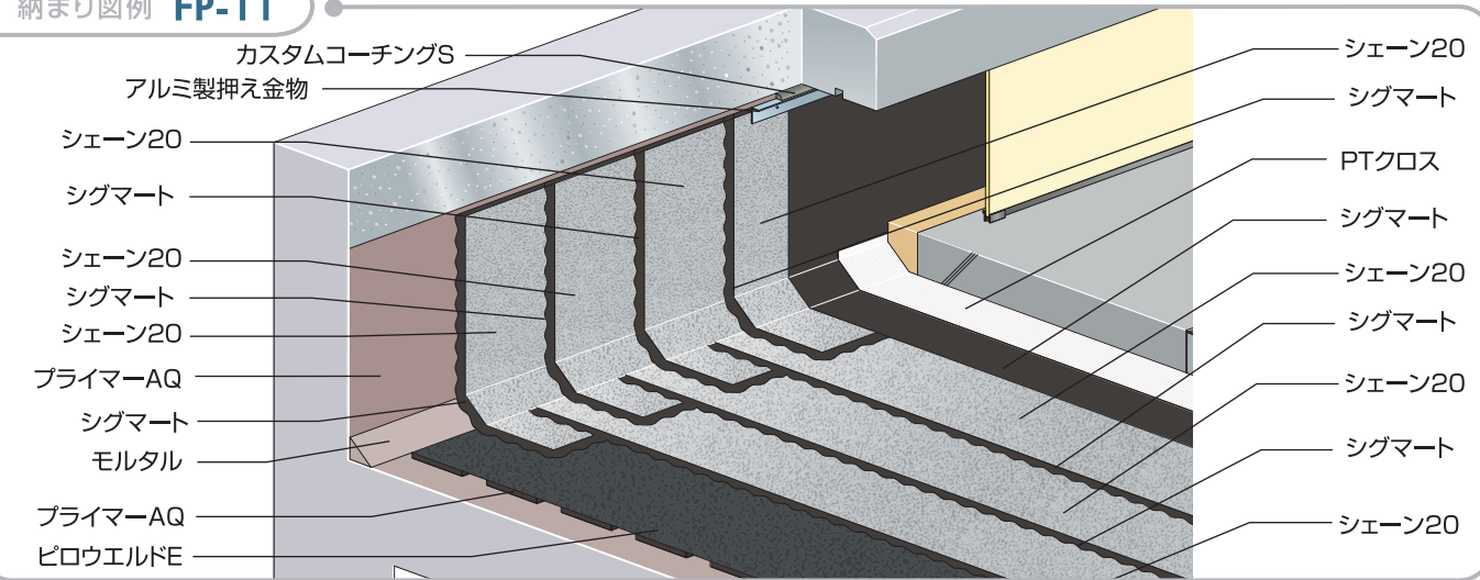
納まり図例 FP-11
