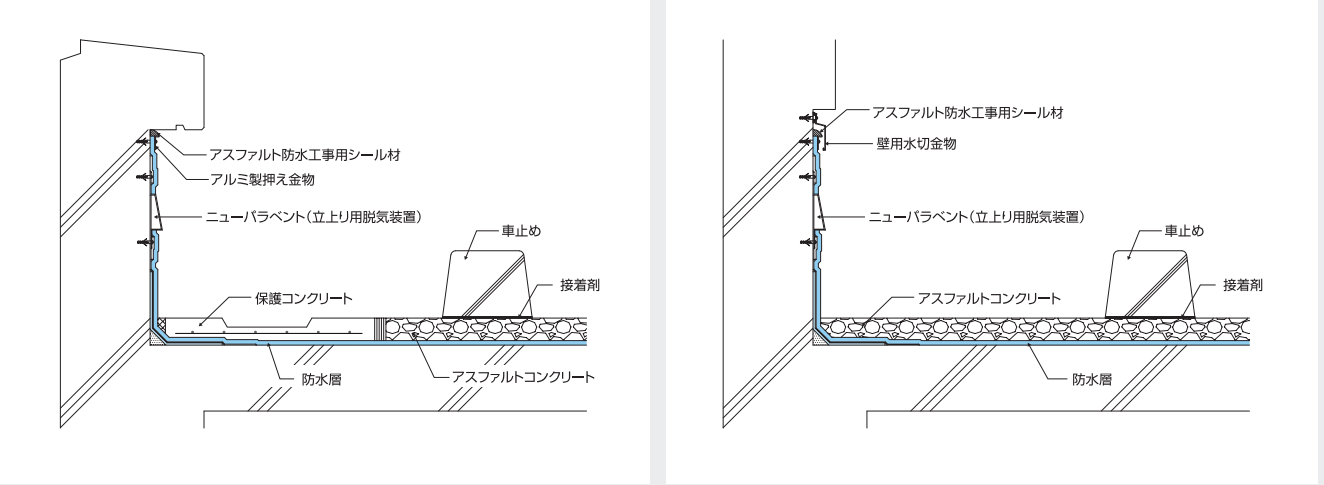
■ピロウエルド新熱工法・改質アスファルト防水熱工法
