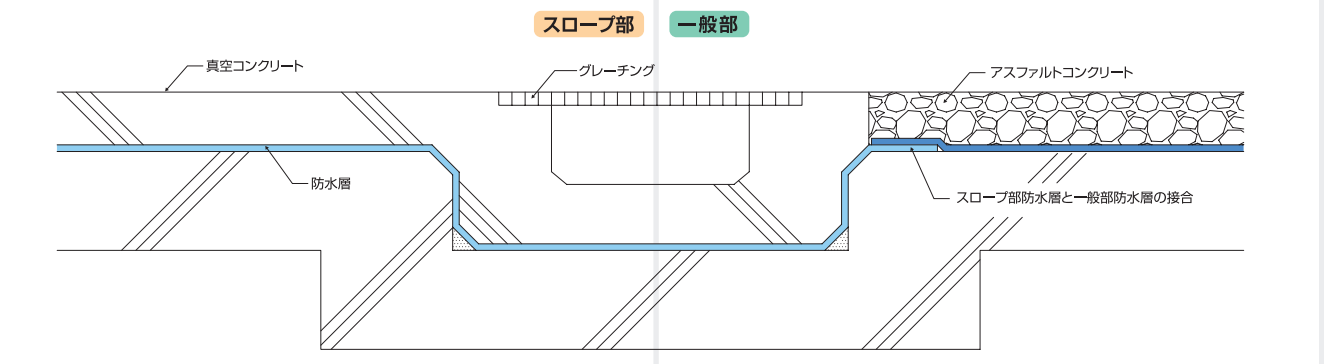
■一般部・スロープ部取合い
