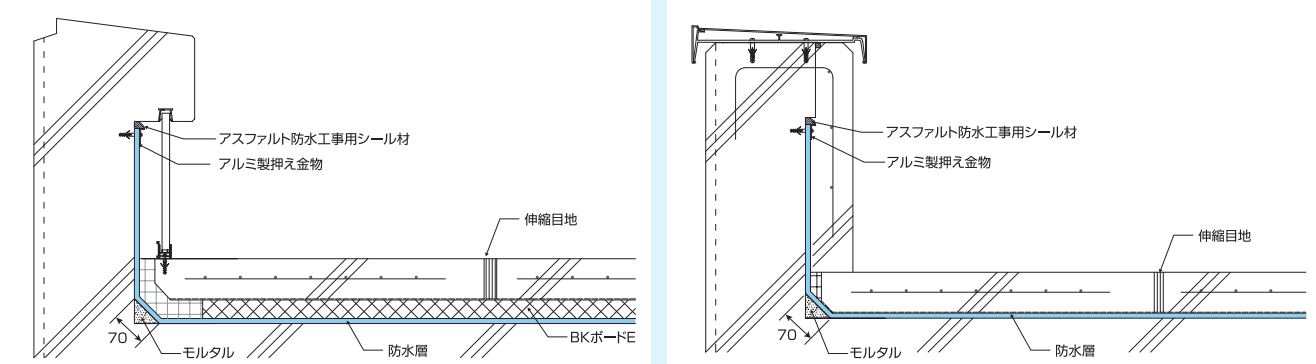
■ピロウエルド新熱工法・シェーン密着工法
