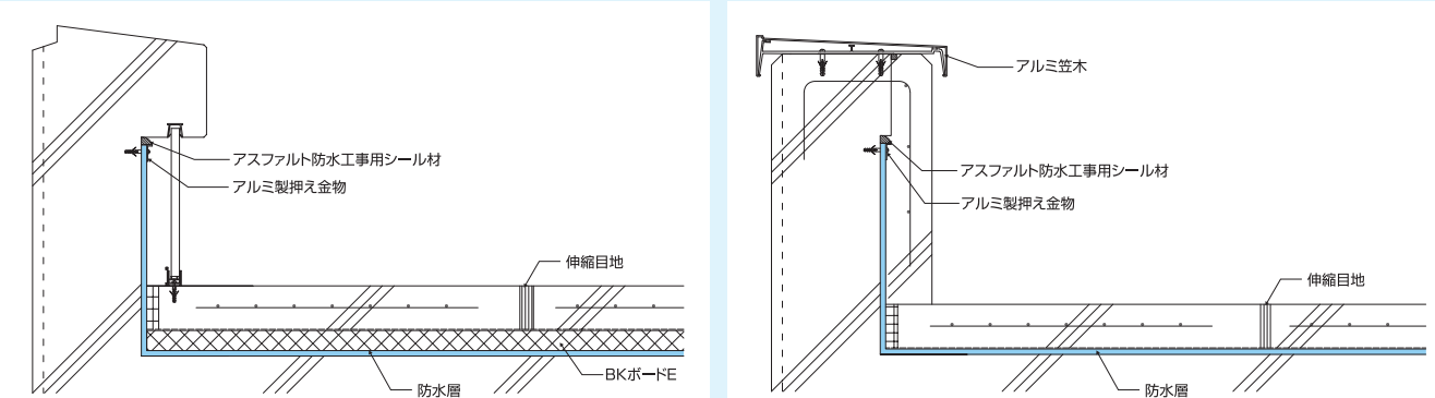
■クリンアス工法・アスオーブ工法・ベストーチ工法
