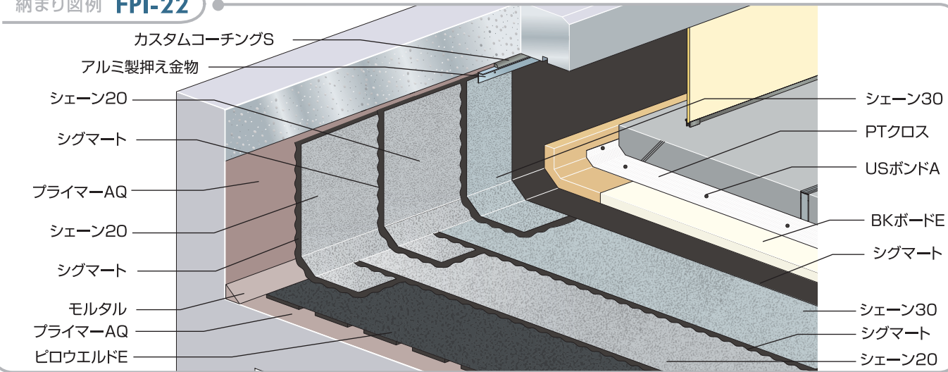
納まり図例 FPI-22
