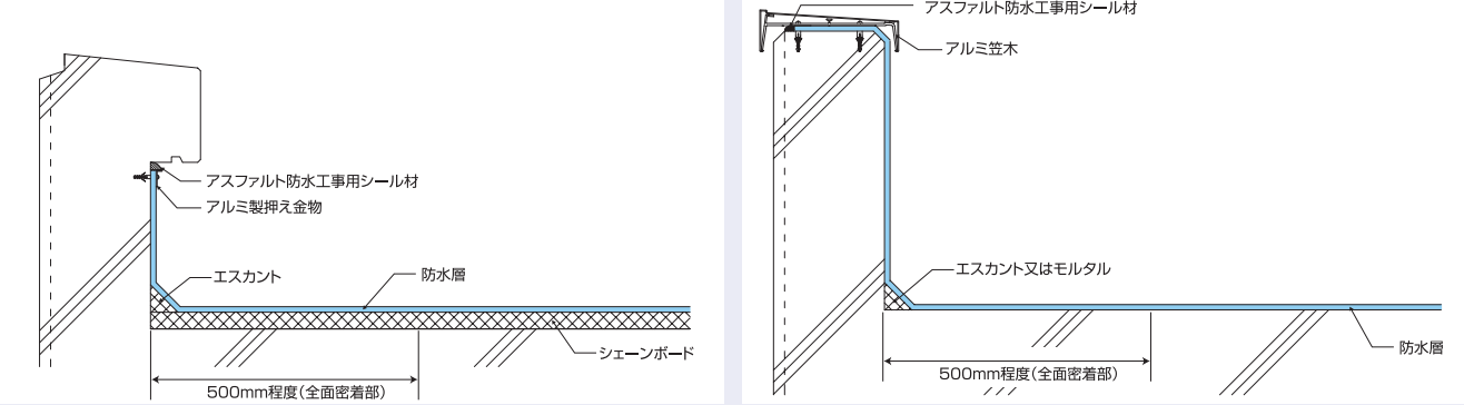
■ピロウエルド新熱工法 (防水工事用アスファルトを使用する工法)
