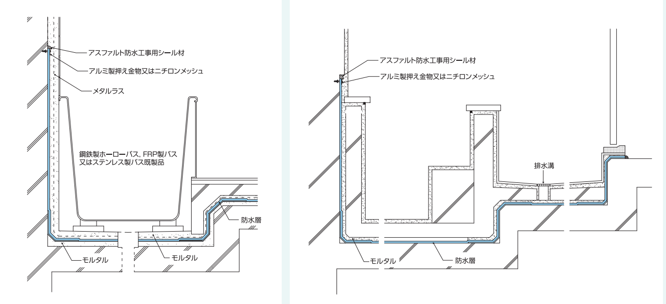
■クリンアス(NEO)工法・アスオーブ工法・(改質)アスファルト防水熱工法
