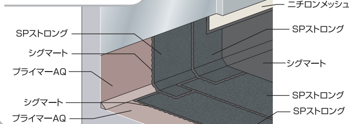
納まり図例 RA-100
