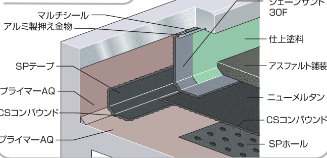
納まり図例 CA-10
