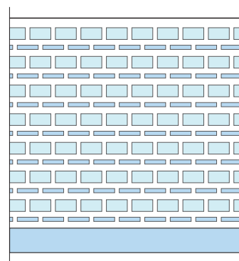
部分粘着層付改質アスファルトルーフィング (粘着層のパターン)
