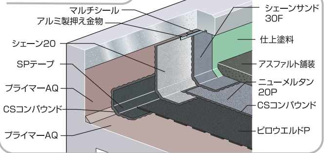
納まり図例 CP-15
