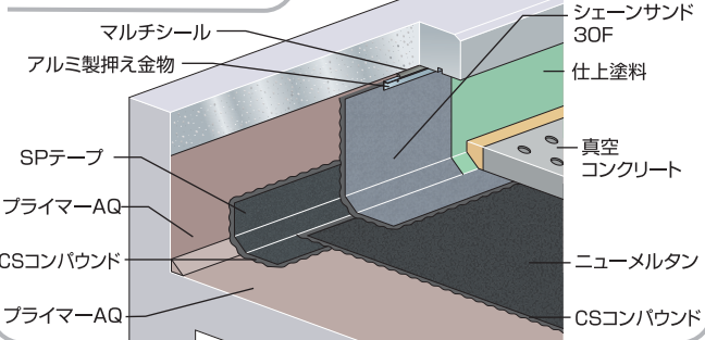
納まり図例 CA-21
